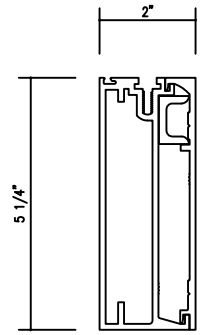
D1 1 DETAIL BOX PERIMETER BP253/BP252
